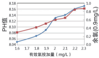
图9 投加次氯酸钠后PH值变化曲线
