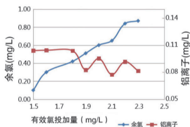
图10 投加次氯酸钠后余氯和铝离子浓度变化曲线
