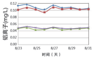
图11 水厂生产过程铝离子检测曲线
